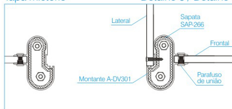
Tapa mictório
